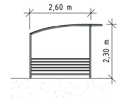
CYKELGARAGE GAVEL 2
