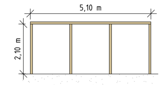
PERGOLA LÅNGSIDA 1
