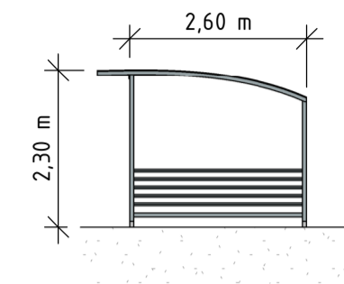
CYKELGARAGE GAVEL 1
