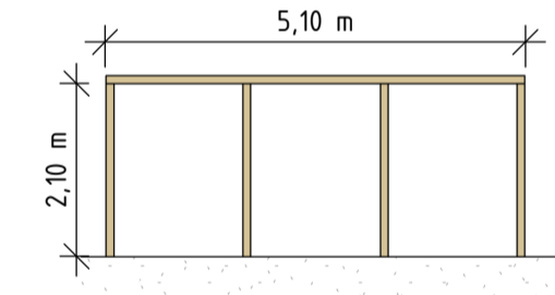
PERGOLA LÅNGSIDA 2
