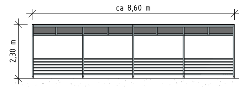
CYKELGARAGE FRAMSIDA
