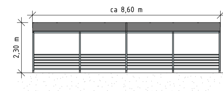
CYKELGARAGE BAKSIDA
