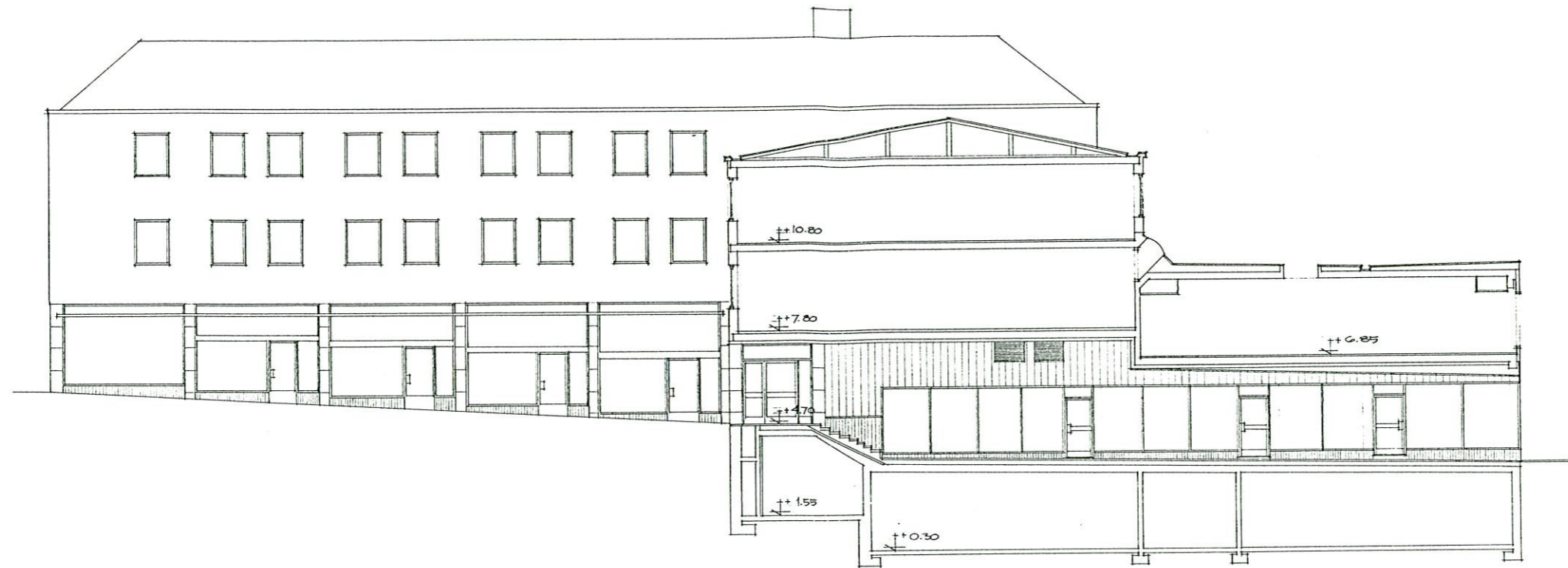
FASAD MOT VÄSTER (TORGET)
