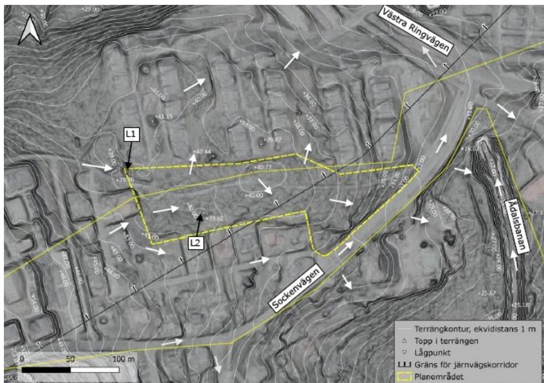
Figur 9 Topografi inom planområdet och omgivningen. Pilarna visar lutningsriktning och gul linje höjdryggar. (Ramboll 2025)
