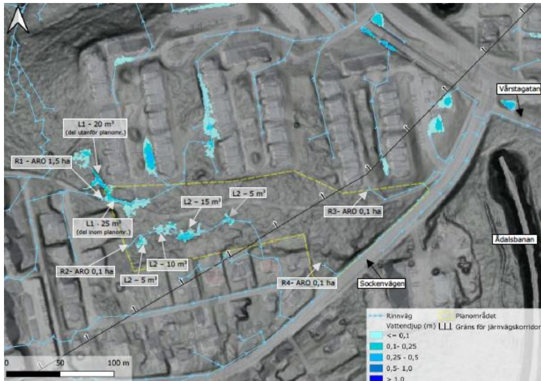
Figur 7 Lågpunktskartering för planområdet vid befintlig situation (Scalco Live, Ramboll 2025).
