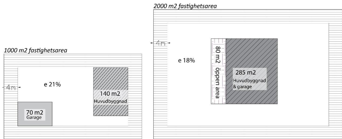
Figur 20. (TV) Illustration över den största tillåtna byggnadsarean av en fastighet om 1000 m 2 . (TH) Illustration över den största tillåtna byggnadsarean av en fastighet om 2000m 2 .
