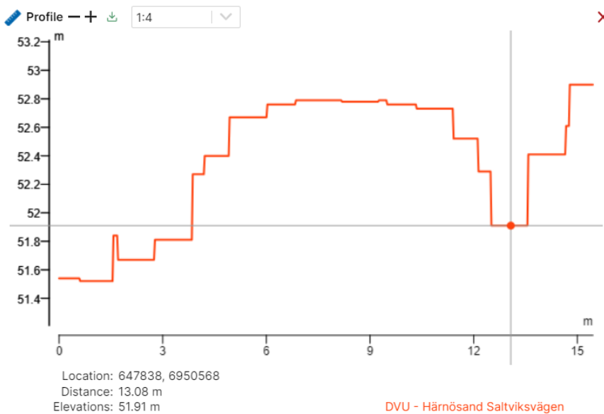
Figur 10. Ungefärlig höjd på vattengång i Trumma B markerad med röd punkt på nivån +51,91 m (RH2000). Profilen sträcker sig i syd-nordlig riktning och korsar Saltviksvägen (Scalco Live, 2024).
