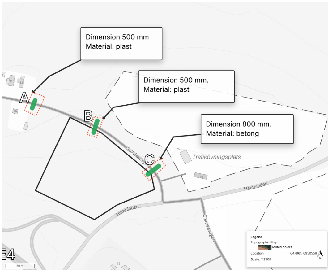
Figur 9. Befintliga dagvattenstrummar markerad med gröna linjer (Trafikverket, 2024). Planområdet markerat med svart linje.
