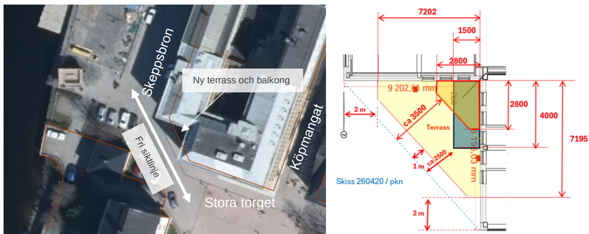
Figur 16. (TV) Fri siktlinje från Stora torget mot vattnet och Nattviken. (TH) Principskiss mått för hörnbalkong och terrass.
