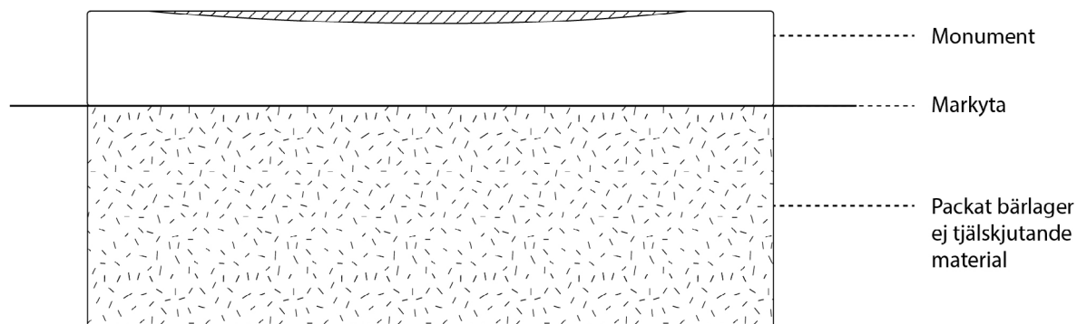
Principskiss för montering
